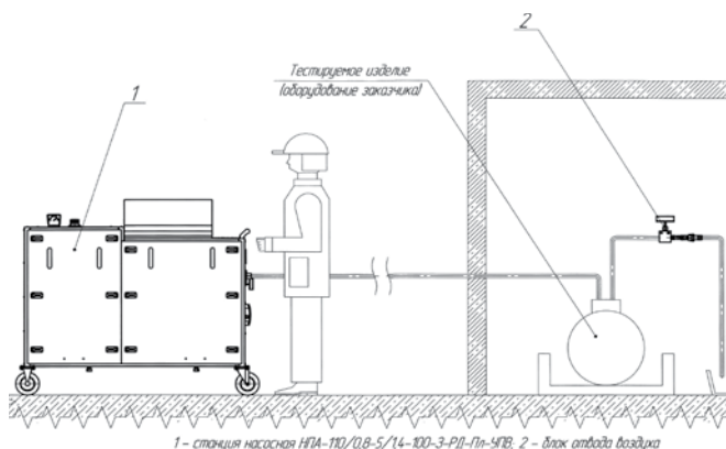
1 - станция насосная НПА-110/0,8-5/1,4-100-3-РП-ПН-5ПБ, 2 - блок отвода воздуха
